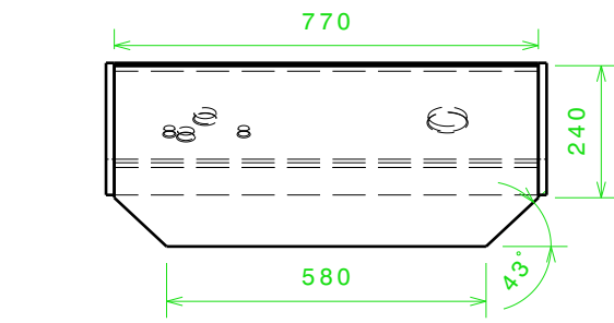
Draufsicht Maßstab: 1:15
