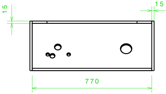
Vorderansicht Maßstab: 1:15
