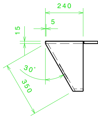
Seitenansicht links Maßstab: 1:15
