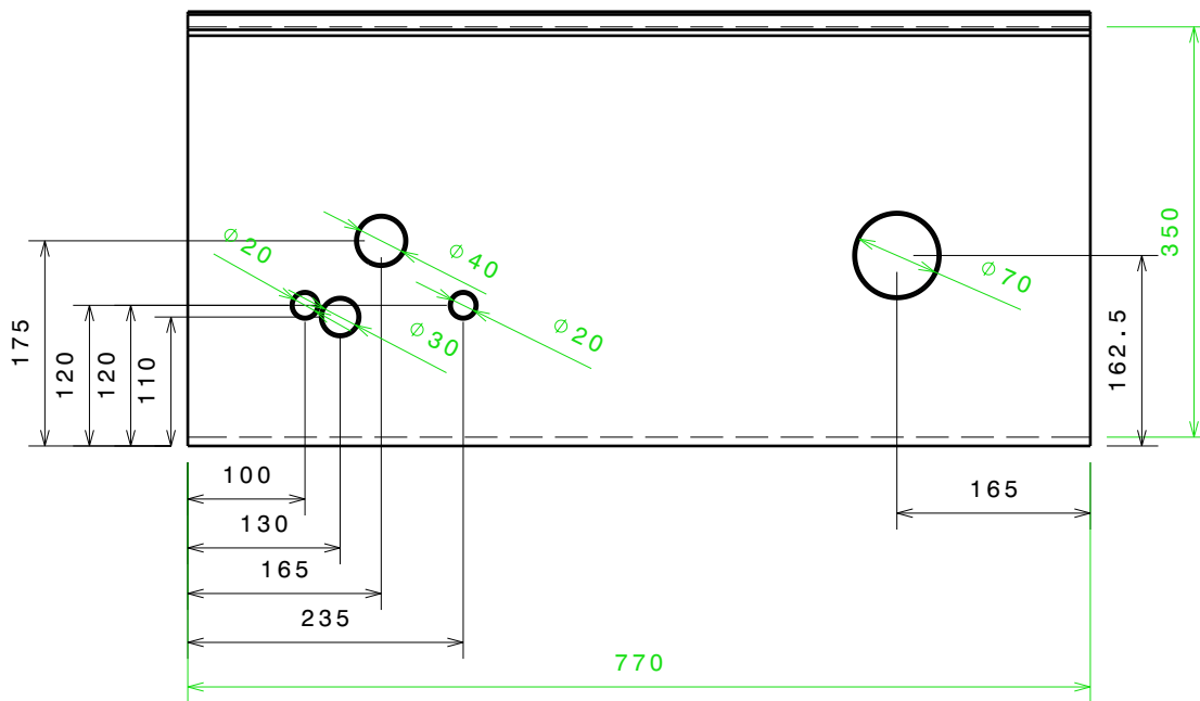
Vorderansicht Maßstab: 1:7
