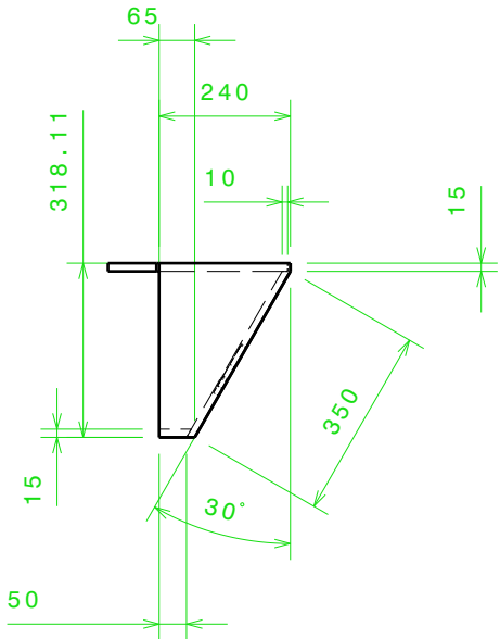
Seitenansicht rechts Maßstab: 1:15
